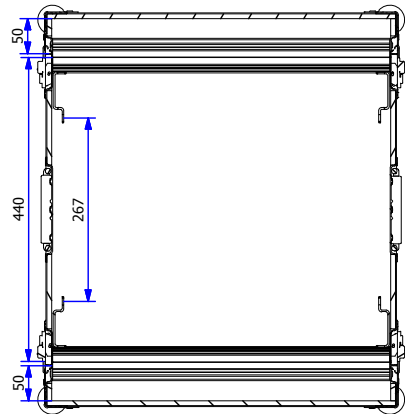
A-A (1 : 11)
