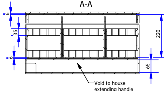
A-A
